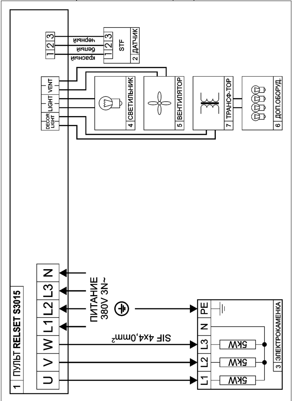
Рис.6 Схема электрическая RELSET S3015 (380В).
