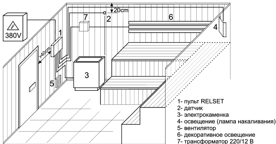
Рис.1 Рекомендуемая схема размещения оборудования.
