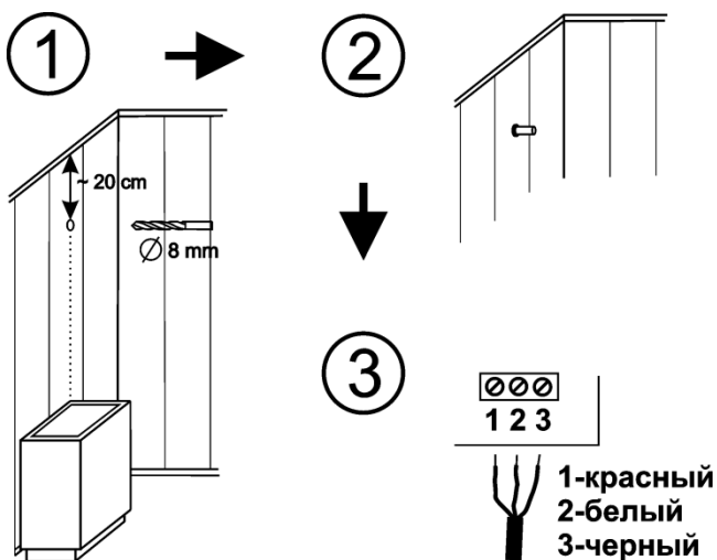
Рис. 3 Монтаж датчика.
