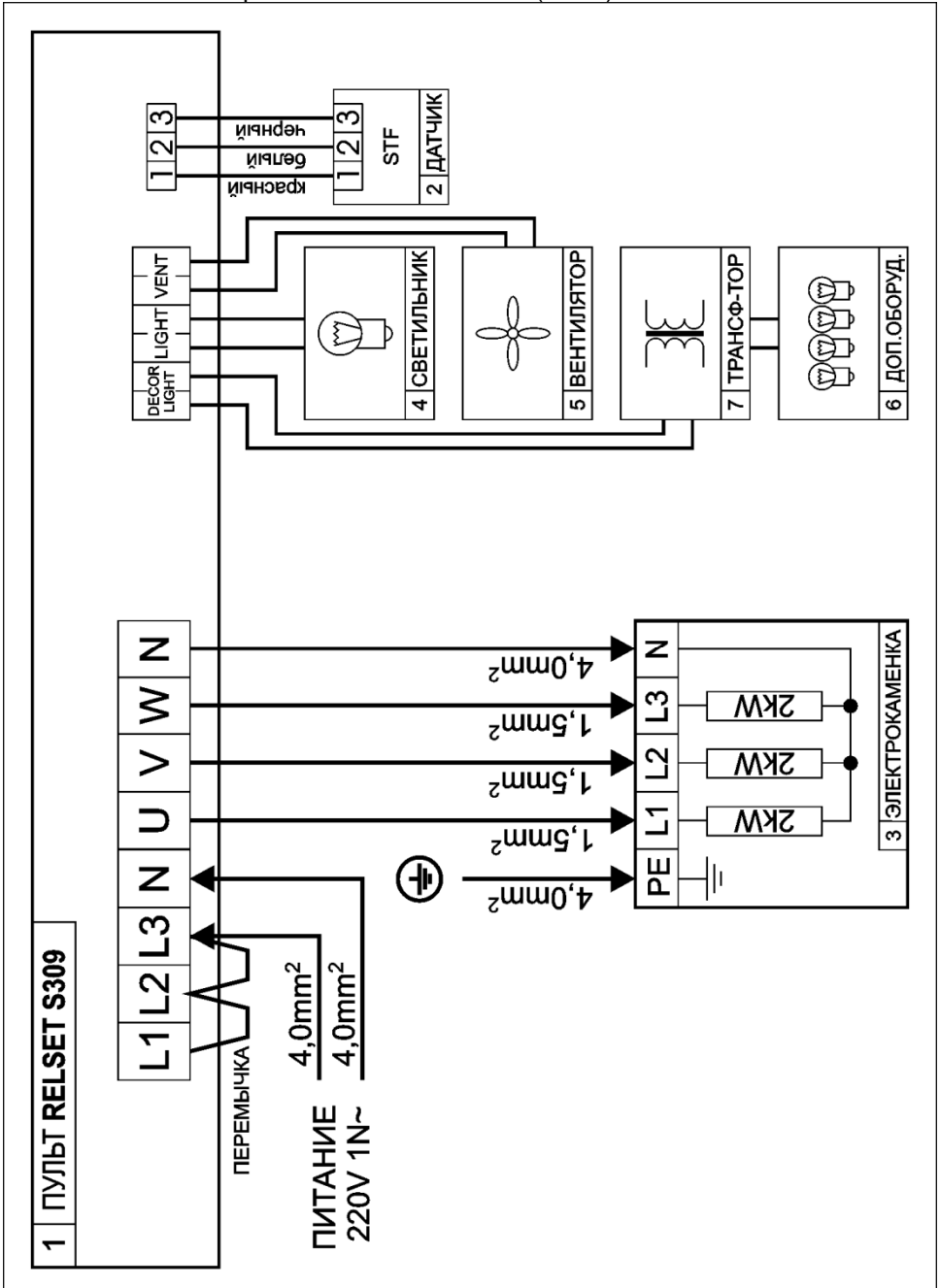
Рис.5 Схема электрическая RELSET S309 (220В).
